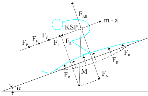
Abb. 2.23: Kräftesystem in der Einwirkung auf den Skiläufer beim Abfahren
